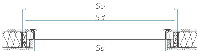
drzwi HARMONY INVEST ODW (otwierane do wewnątrz)
