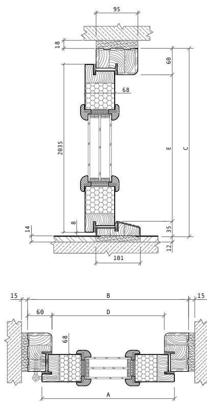
Drzwi szklone z ramką PCV
