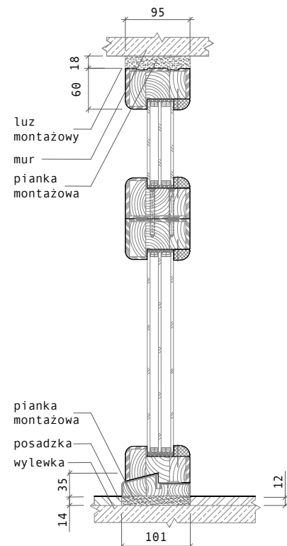
Przekrój przez dostawkę boczną
