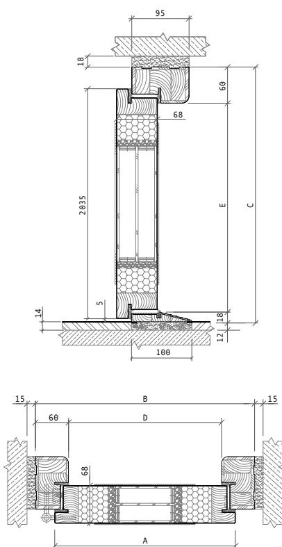
Drzwi szklone z ramką inox
